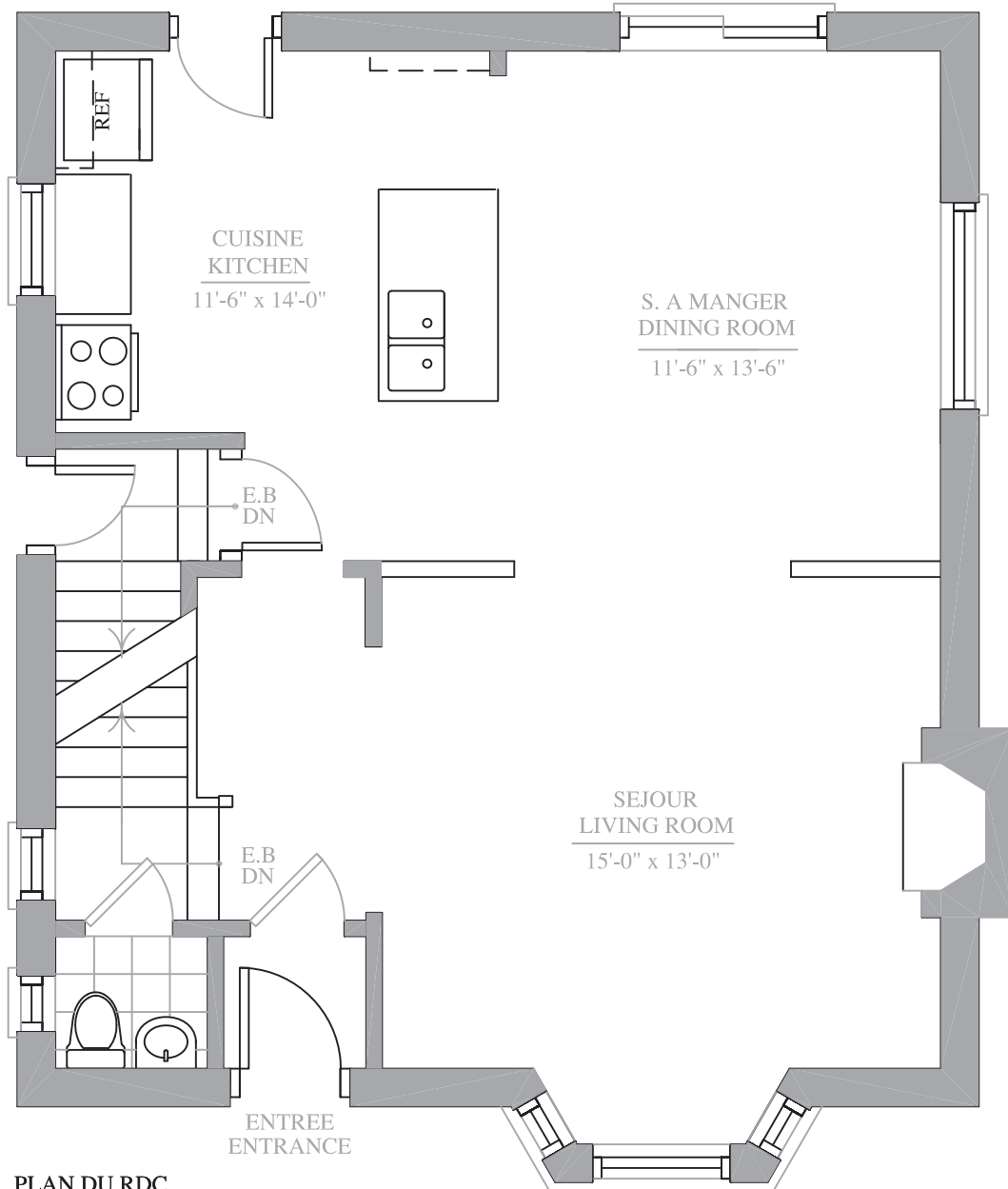
PLAN DU RDC MAIN FLOOR PLAN
